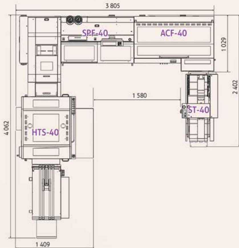
Dimensions de la machine (en mm)
