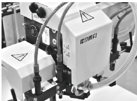
Tête d'alimentation Komfi
